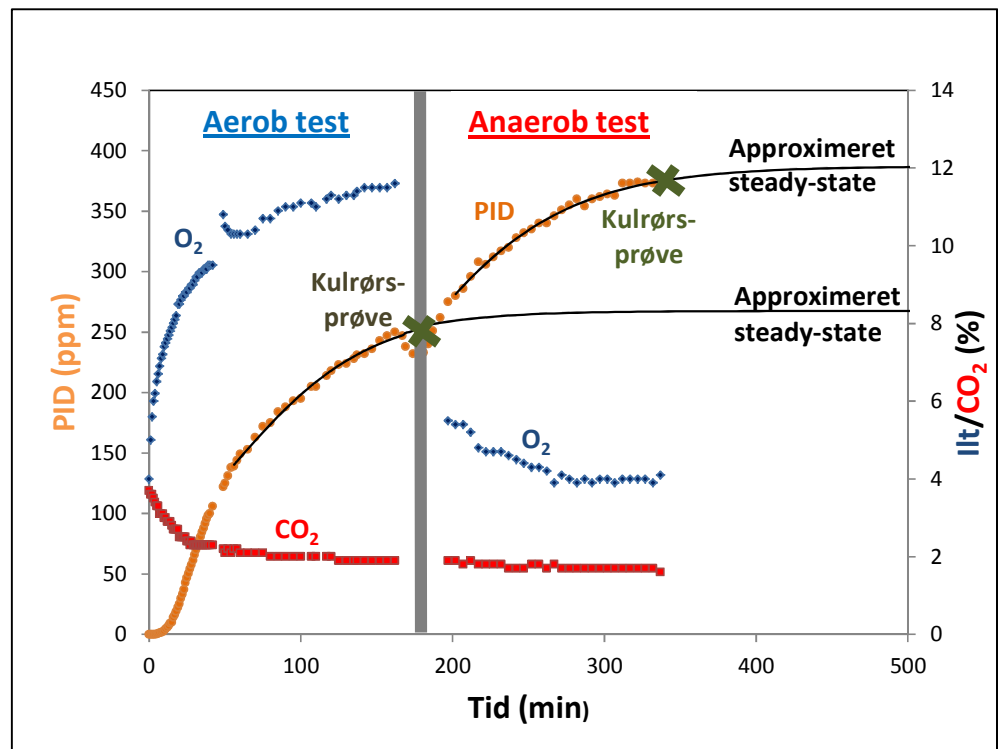
Figur 4.1: Resultater målt i P2: O 2 , CO 2 og PID. Omkring 50 min blev Q ved et uheld momentant opjusteret til 1,2 L/min, og der ses en stigning af ilt i udløbet (P2). Det aerobe testforløb var ca. 170 min og det anaerobe testforløb var ca. 160 min.
