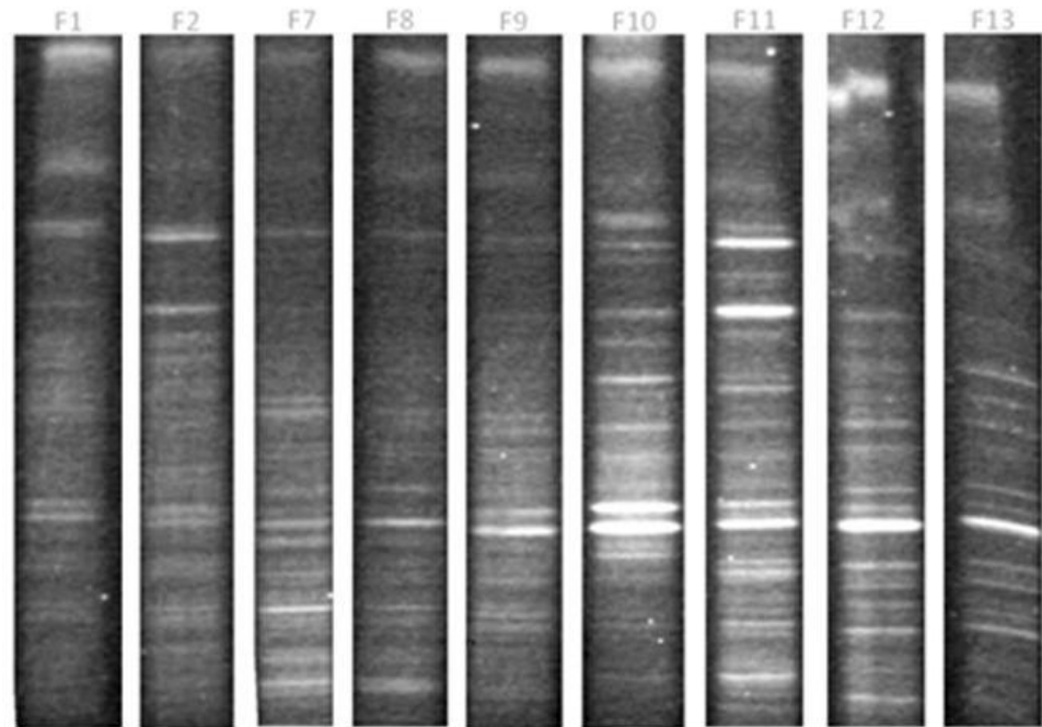
Figur 5.1: DGGE-gel, hvor der er anvendt en generel primer designet til at ramme 16S-rRNA genen for bakterier i jordprøverne (341F/518R primersættet).
