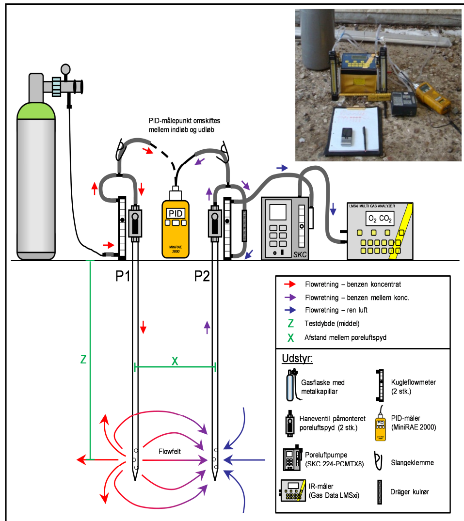
Figur 2.1: Foto og skematisk tegning af feltopstillingen. P1 er injektionspunktet og P2 er opsugningspunktet. Pilottesten er udført i dybden 100 cm (Z) og med 20 cm afstand mellem poreluftspydene (X).
